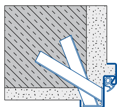
Montāža mūra sienās ar enkuriem
