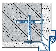
Montāža ar dziļju enkuriem
