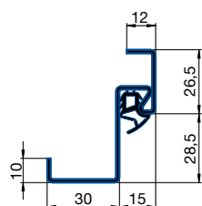
Standarta stūra kārba
