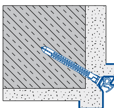
Speciālā stūra kārba Montāža ar dziļju enkuriem caur kārbu
