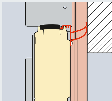
Упор перемычки с ThermoFrame
