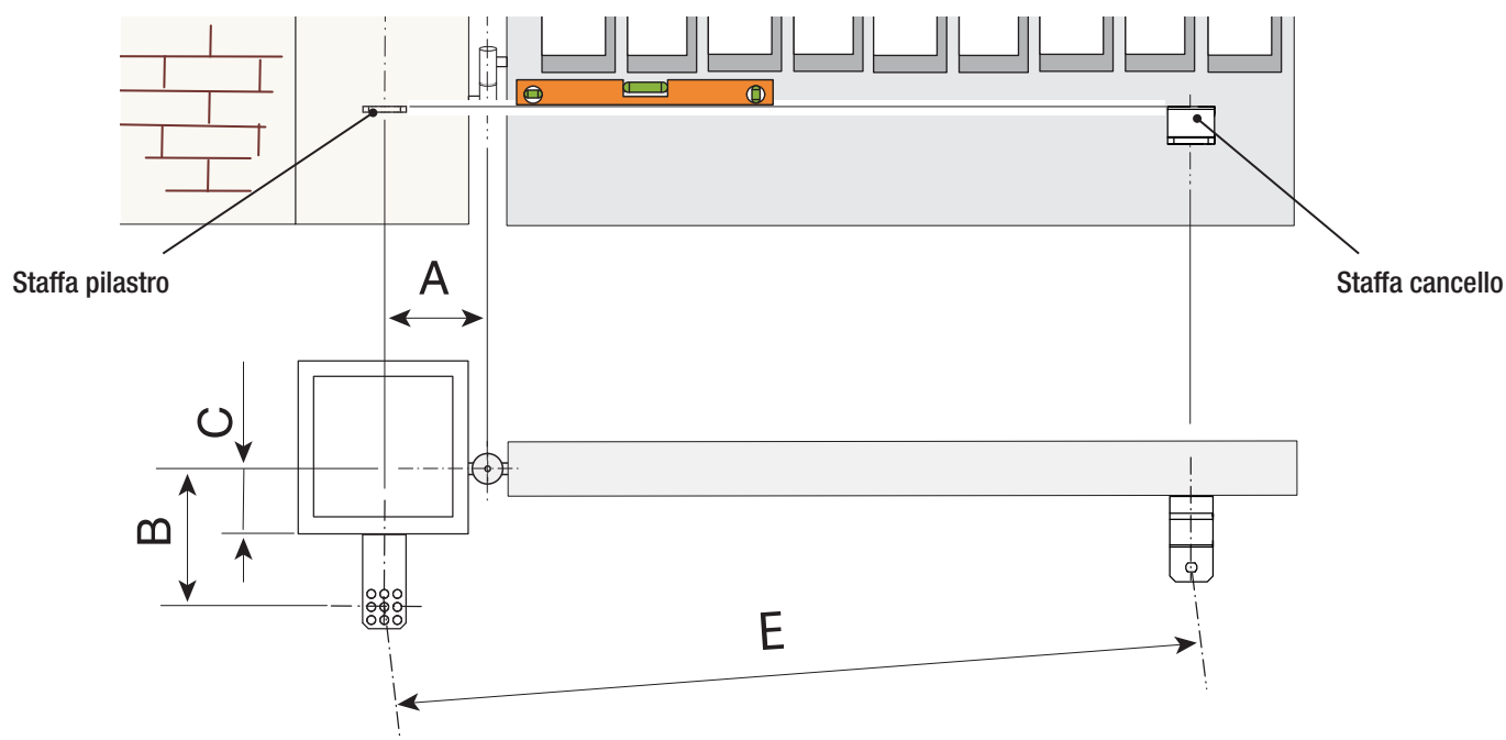
Dimensioni applicazione (mm)
